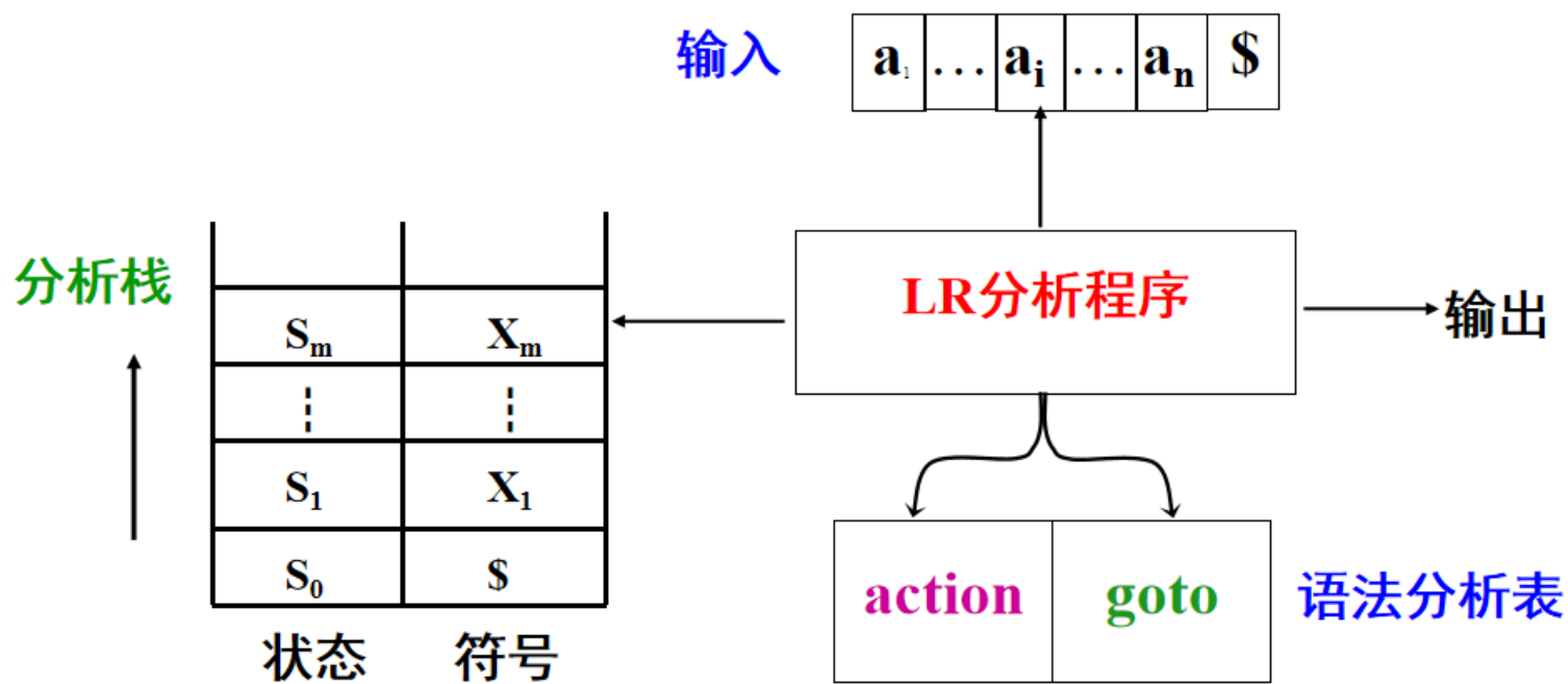
LR分析器的模型
